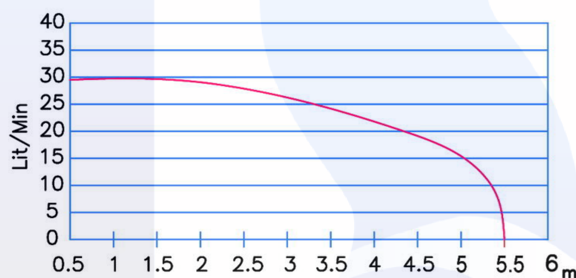
منحنی دبی-ارتفاع
