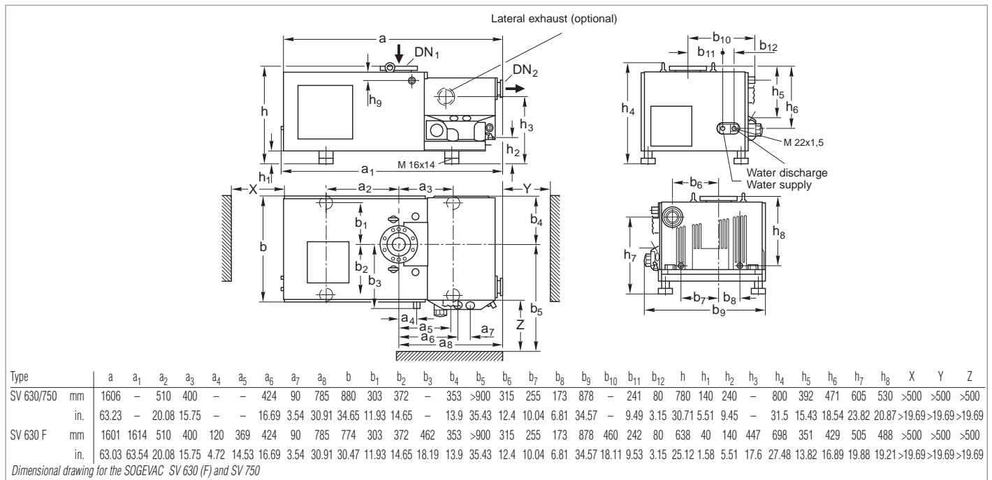
SOGEVAC SV 630
