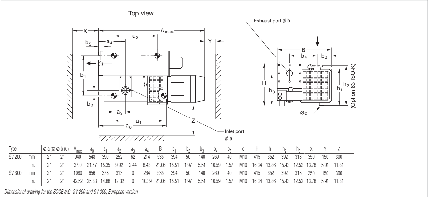
SOGEVAC SV 300
